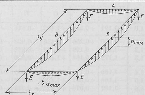
Tafel I. Gesamtauflegerdrücke und Scheitelwerte der Auflagerdrücke rechteckiger Platten infolge gleichmässig verteilter Belastung (Querdehnung \nu = 1/6 )
