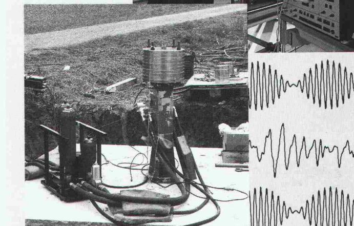
Schwingungserregung einer Fundamentplatte.
