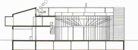
Schnitt Hof
