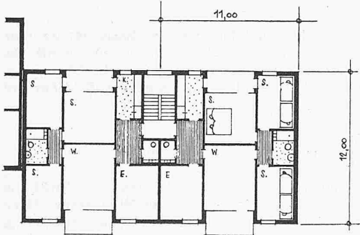
FÜNZZIMMERWOHNUNG, DREI GESCHOSSIG (SCHEMA ORANGE)
