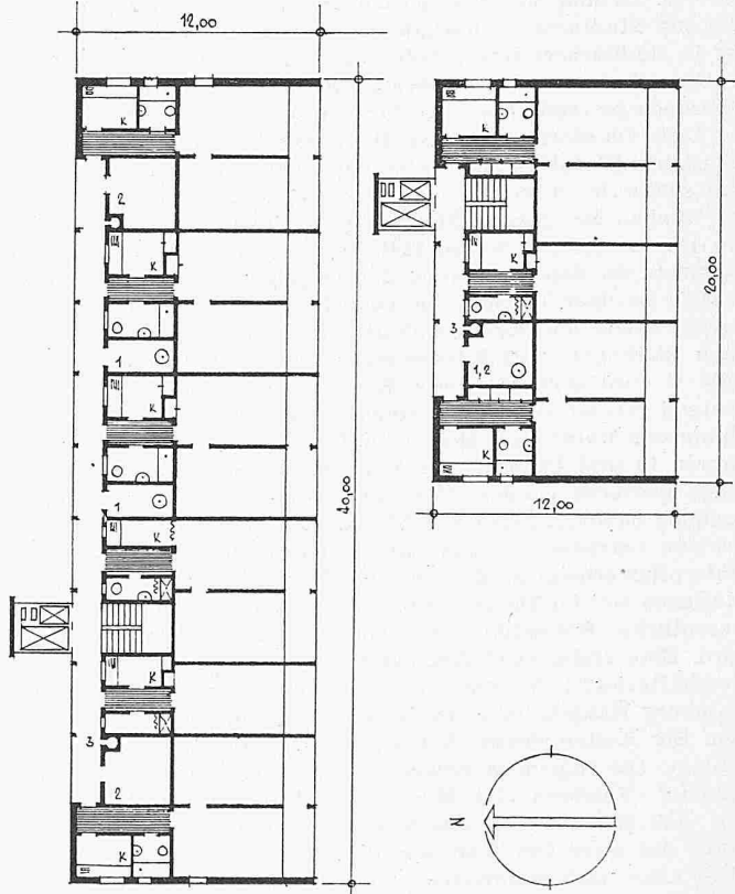
LAUBENZANGHAUS 14 WOHNGESCHOSS, PRO GESCHOSS 1 EINZIM. + 5 ZWEIZIM.
