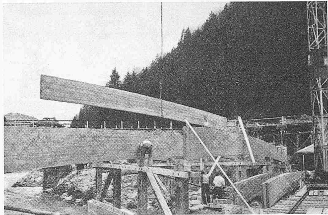
Bild 9. Ponte Sordo, Lehrgerüst aus Hetzertträgern
