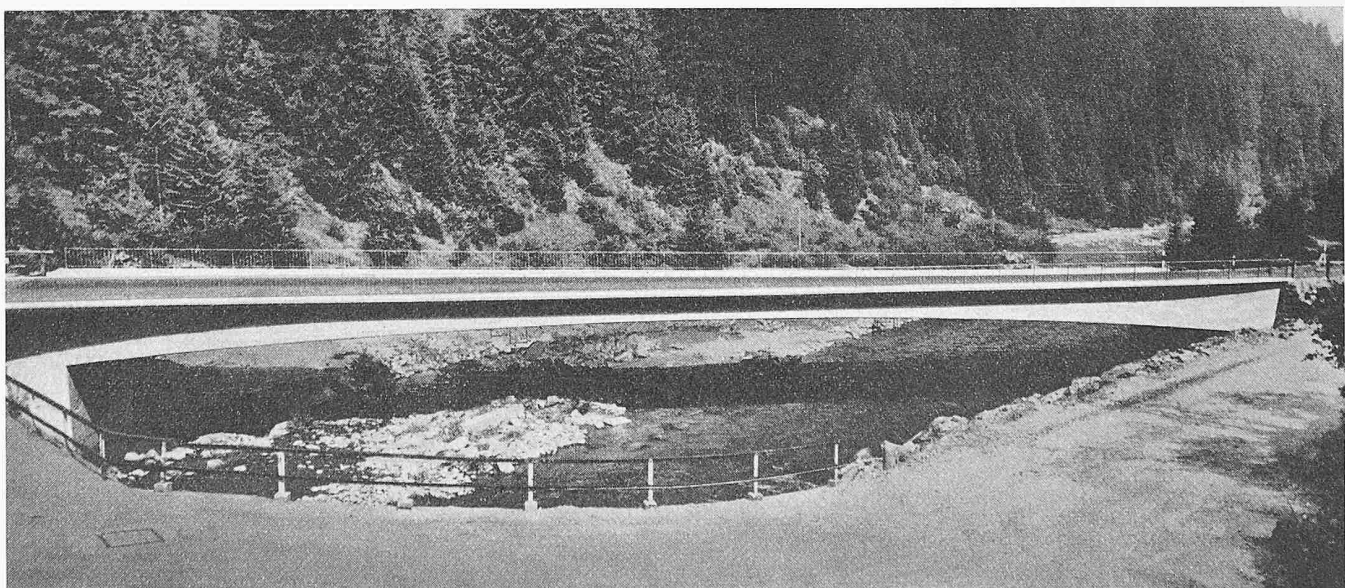
Bild 1. Ponte Sordo, Ansicht aus Südwesten, Oberstromseite, vorn links die alte Brücke
