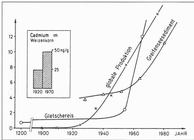
Bild 1. Cadmiumproduktion und -konzentration in Funktion der Zeit. Globale Cd-Produktion in 10^3 t/Jahr; Gletschereis in \mu\text{g}/\text{kg} ; Sediment (Greifensee) in \text{mg}/\text{kg} ; Weizenkörner in \mu\text{g}/\text{kg}
