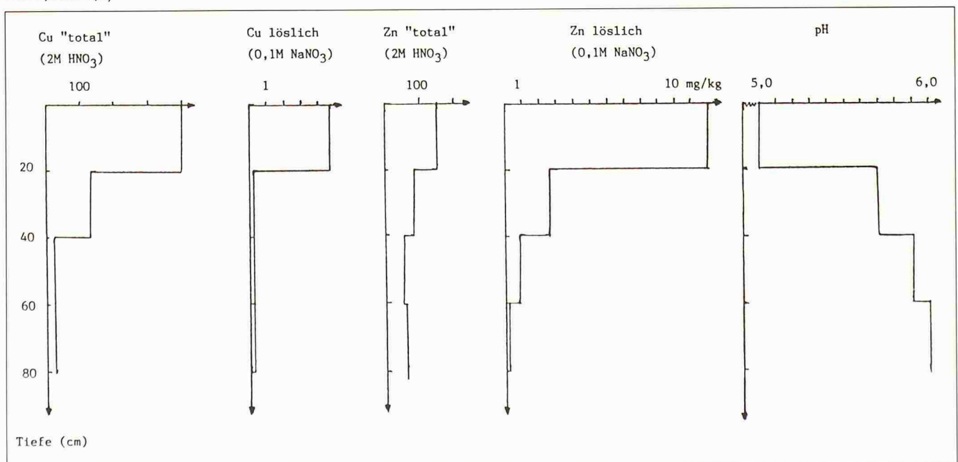
Bild 5. Verteilung von totalem sowie löslichem Kupfer und Zink im Profil eines belasteten sauren Bodens (pH innerhalb des Profils von 5,0 bis 6,0)
