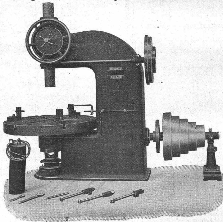
Riemenscheiben-Ausbohrmaschine.
