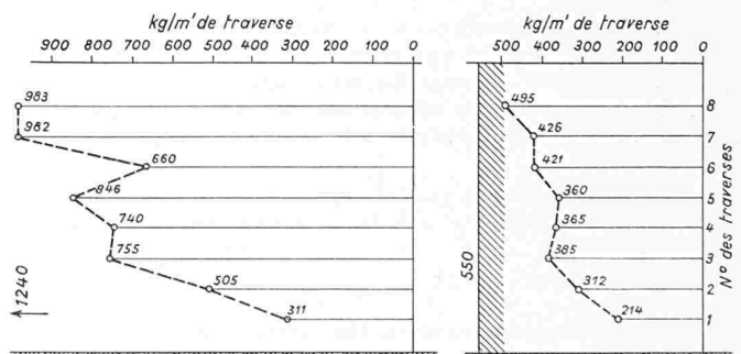
Fig. 3b. Tablier latéral. A gauche pressions S normales au tablier; à droite pressions Q tangentielles au tablier
