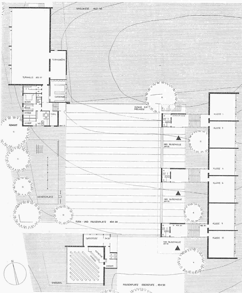
Erdgeschoss 1:700
