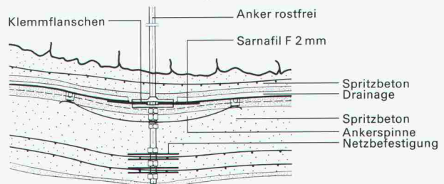
Aufbau der Tunnelabdichtung mit Sarnafil F 2 mm im Verzweigungsbereich bei ständig wechselndem Querschnitt.
