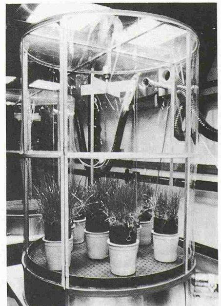
Expositionsanlage für Pflanzenversuche: In Pflanzenkammern werden Graskulturen katalysierten Automobilabgasen ausgesetzt, um zu untersuchen, ob sich in oder auf den Pflanzen Platin abgelagert. (Bild: Fraunhofer Institut ITA)
