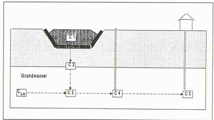
Bild 4. Messstrategien zur Ermittlung der Endlagerqualität
