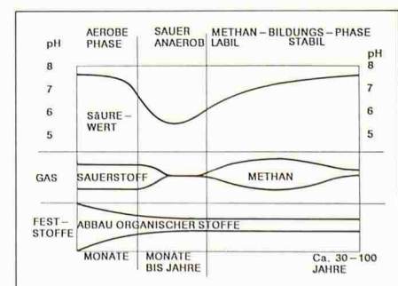
Bild 2. Die Entwicklungsphasen einer Reaktordeponie
