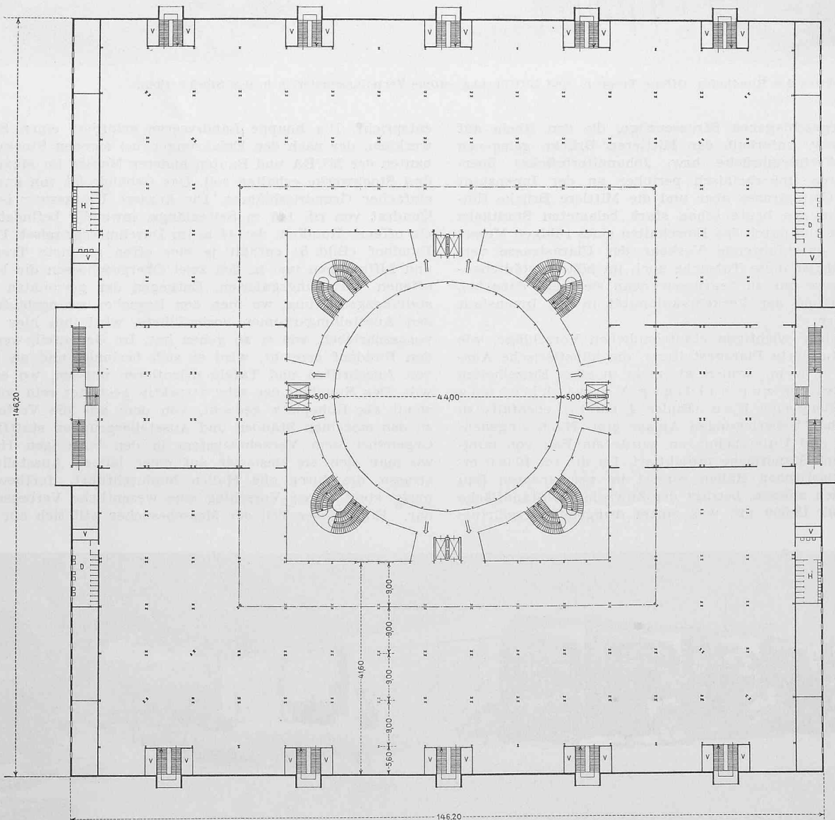
Bild 9. Obergeschossgrundriss, 1:1000. V = Ventilationschacht.
