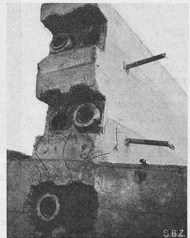
Bilder 26 und 27. Stadion Wankdorf in Bern. Tribünenträger von 36 m Spannweite als Träger für vorkragende Zylinderschalen, Vorspannkraft pro Träger 12 \times 80 = 960 t. Rechts Vorspannarmierungen zum Teil schon gespannt. Projekt: Ing.-Bureau Hartenbach & Wenger, Bern.
