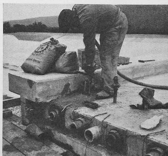
Bilder 21 und 22. Brücke über den Oberwasserkanal des Kraftwerks Wildeg-Brugg, rechts Injektion der Vorspannarmierungen, Vorgespannte kontinuierliche Massivplatte, Spannweiten 19,5 + 24,0 + 19,5 m, Plattenstärke in Feldmitte 0,40 m, totale Vorspannkraft 660 t. Projekt: Ing. E. Schubiger, Zürich.
