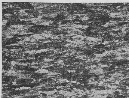
Bild 14. Mikrogefüge des patentierten, gezogenen Stahldrahtes
