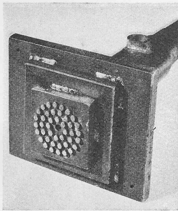
Bild 9. Fester Hauptanker für 42 Drähte \phi 5 mm
