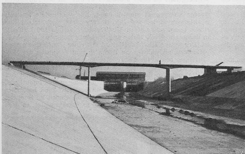
Bilder 21 und 22. Brücke über den Oberwasserkanal des Kraftwerks Wildeg-Brugg, rechts Injektion der Vorspannarmierungen, Vorgespannte kontinuierliche Massivplatte, Spannweiten 19,5 + 24,0 + 19,5 m, Plattenstärke in Feldmitte 0,40 m, totale Vorspannkraft 660 t. Projekt: Ing. E. Schubiger, Zürich.
