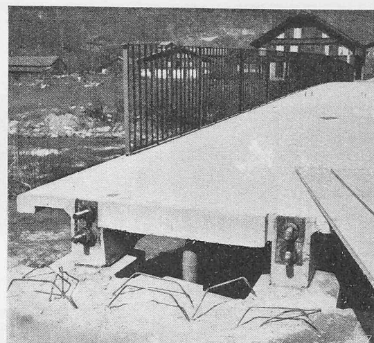
Bilder 17 und 18. Aaresteg bei Innertkirchen, Kontinuierlicher Plattenbalken, Spannweiten 11,5 + 19,5 + 11,5 m, Trägerhöhe in Feldmitte 0,48 m, Vorgespannt mit 4 Kabeln mit je 60 t Vorspannkraft, Projekt: Obering. J. Bächtold, Innertkirchen und Ing.-Bureau M. R. Ros, Zürich
