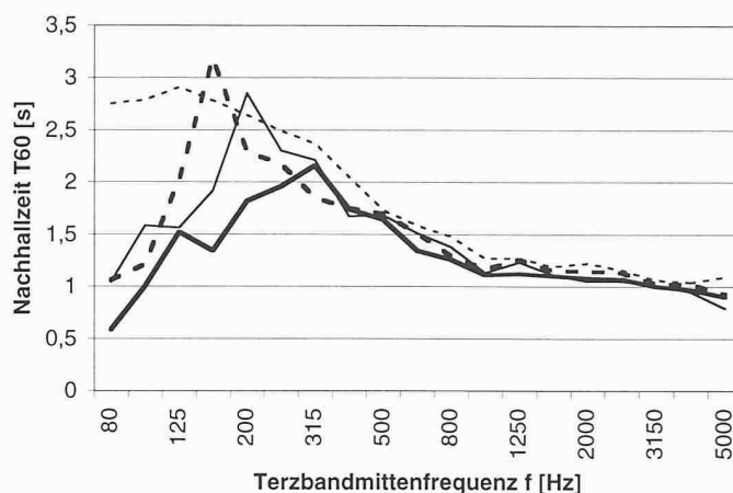
Einfluss der Leichtbauwände auf die Halligkeit
