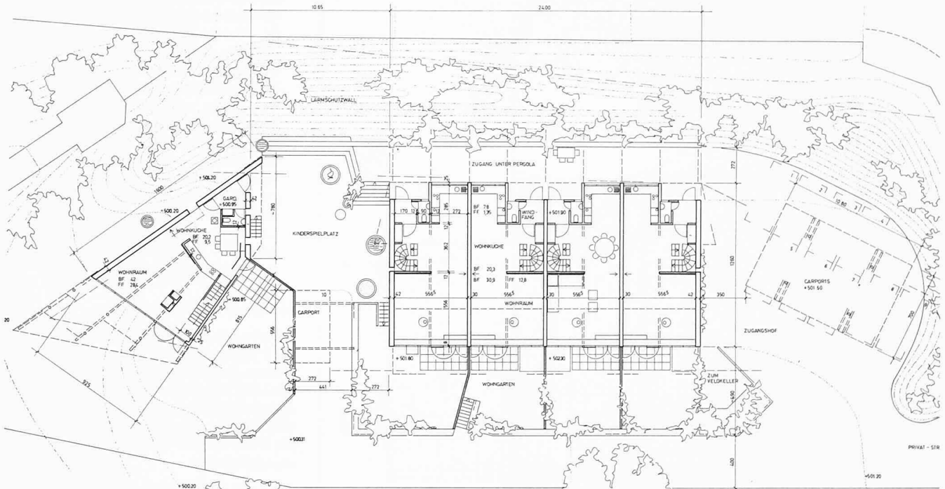
Grundriss, Erdgeschoss
