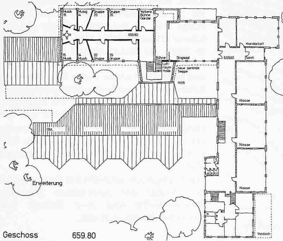
Grundrisse, Schnitte, Ansichten 1:900
