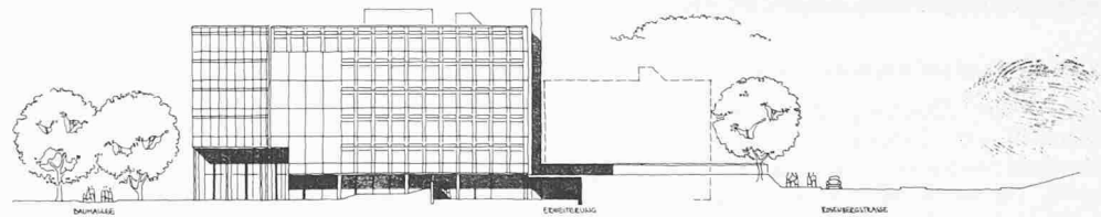
Ansicht von Osten 1:1000
