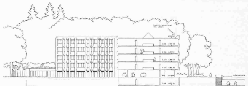
Schnitt Halle 1:1000
