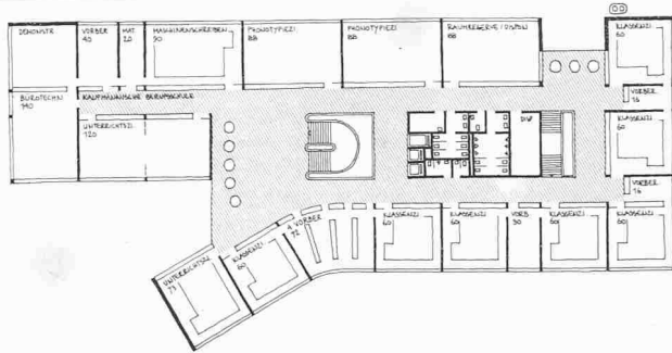
Grundriss 3. Obergeschoss 1:1000
