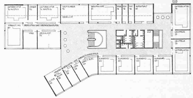
Grundriss 4. Obergeschoss 1:1000
