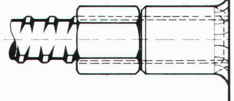
Gewi-Anschluss im Stahlbau
