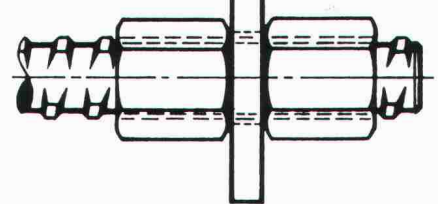
Gewi-Endverankerung
