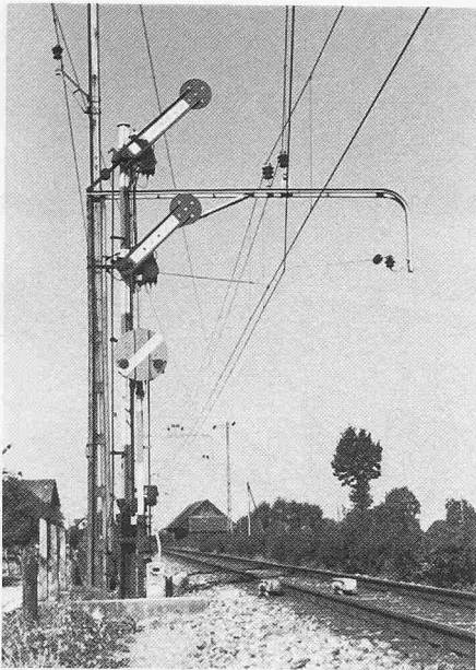
Bild 1. Zweiflügliges mechanisches Hauptsignal mit mechanischem Durchfahrtsignal
