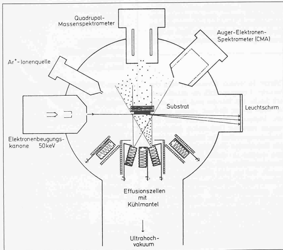
Schematische Darstellung des Prinzips der Molekularstrahl-Epitaxie: Im Ultrahochvakuum wird das aus getrennten Öfen, den Effusionszellen (unten), verdampfte Material auf eine Unterlage, das Substrat, in nur wenigen Atomlagen gezielt abgeschieden. Zahlreiche Messgeräte (oben) überwachen dabei bereits während des Wachstums den Aufbau der dünnen Kristallschichten aus Halbleiter-Materialien.
