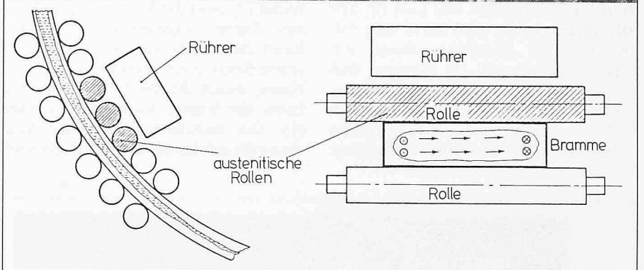
Bild 5. Elektromagnetischer Lineararmrührer in einer Brammenstranggießanlage Oben: Photographie des Segments mit eingebautem Rührer Unten: schematische Darstellung
