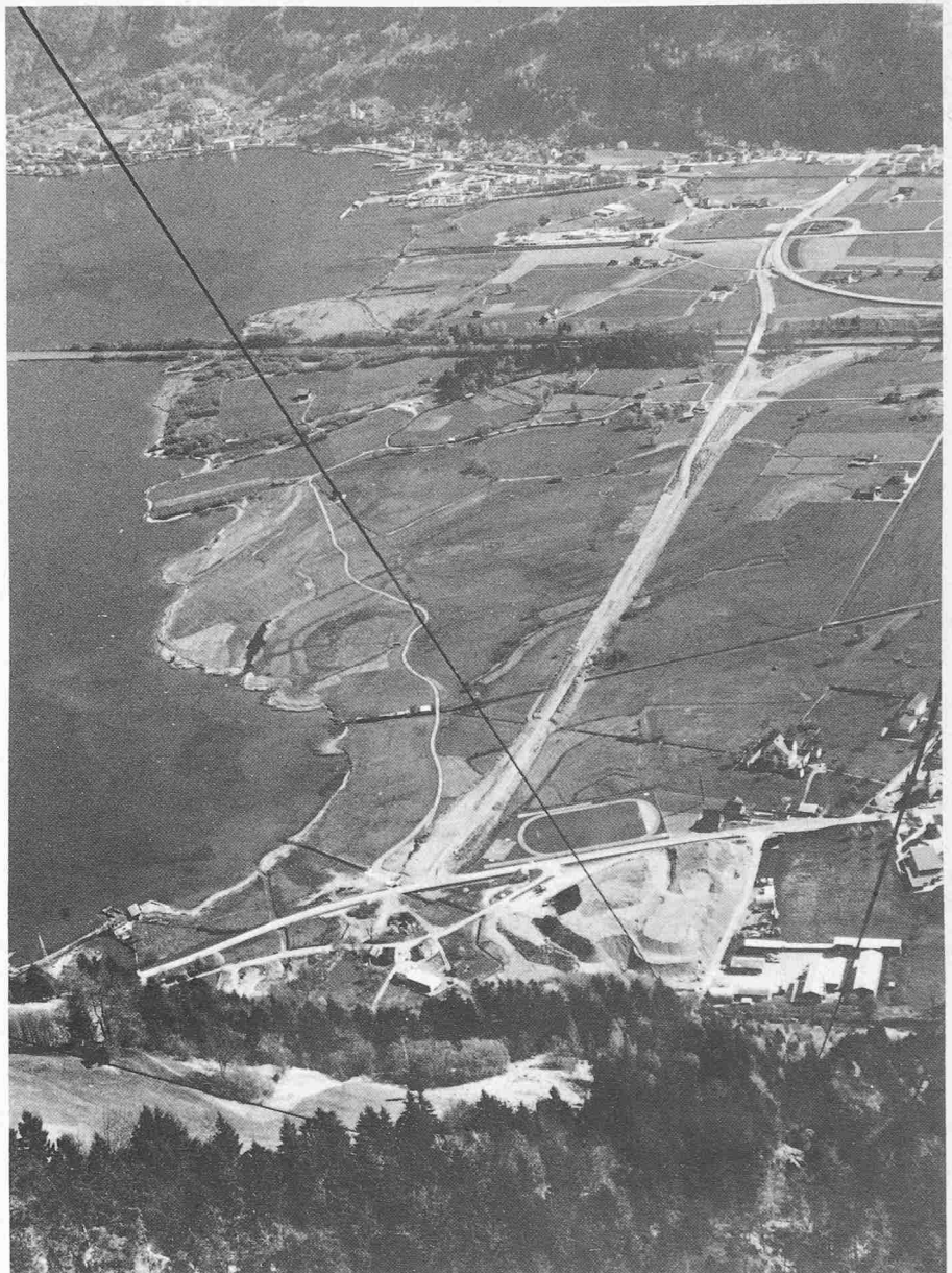
Bild 4. Übersicht Reussebene. Quer durch die Reussebene ist die Baupiste erstellt. Das Autobahnende nördlich von Altdorf wird im Gegenverkehr befahren. Die Bauarbeiten der Autobahnhalfte Flüelen-Erstfeld sind noch nicht begonnen (Mai 1975). Am unteren Bildrand rechts ist das Mannschaftslager des Bauloses Biel des Seelisbergtunnels. Links davon befindet sich der etwa 22 000 m 2 grosse Deponieplatz für das gebrochene Tunnelausbruchmaterial, das als Foundationsschicht des Strassenbelages verwendet wurde. Die Deponie umfasste bis zu 125 000 m 3 und war stellenweise bis zu 10 m hoch
