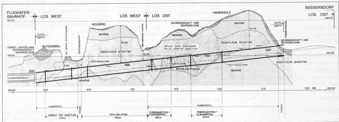
Bild 1. Geologisches Längenprofil mit Eintrag der Dichtungsschirme und der Abdichtungsmassnahmen in der Tunnelsohle
