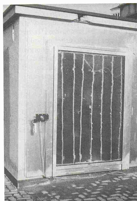
Bild 4. Testkollektor von 2,5\text{ m}^2 Fläche, am Liftaufbau des Amtes für technische Anlagen und Lüfthygiene montiert.
