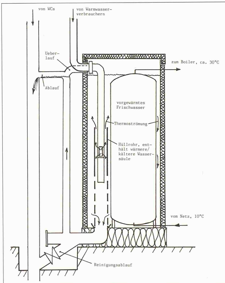
Bild 3. Schema der Abwasser-Wärmerückgewinnung
