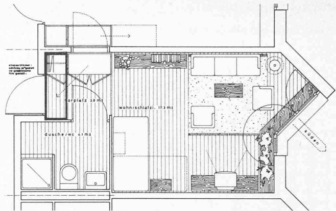
Grundriss eines Pensionärszimmers 1:100
