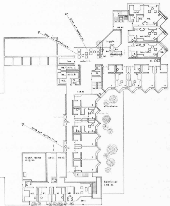
Grundriss 1. Obergeschoss 1:700
