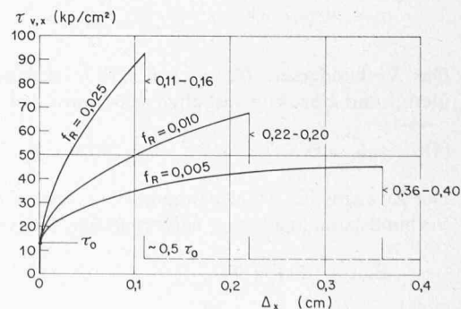
Bild 7. Verbundgesetze \tau_{v,x} = f[\delta_x]
