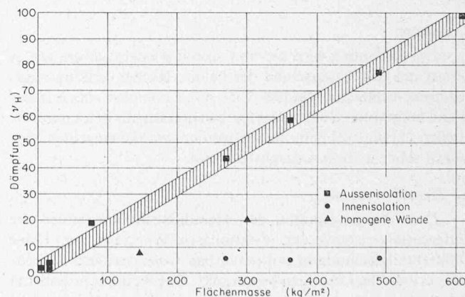
Bild 2. Dämpfung v_H in Funktion der Wandmasse
