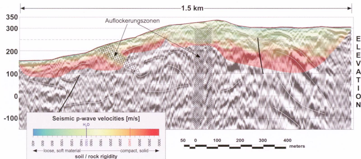
Fig. 4d: Vorschlag einer Interpretation des hybridseismischen Profils in Fig. 4c. Zu beachten ist die an mehreren Stellen gute Übereinstimmung der refraktionstomographisch und reflexionsseismisch abgebildeten Strukturen, z. B. bei der flach einfallenden Auflockerungszone in der linken Profilhälfte. Die visuelle Korrelation ist als gegenseitige Kalibration der beiden Auswertungsverfahren zu betrachten und eine Hilfe bei der geologisch-geotechnischen Interpretation.
