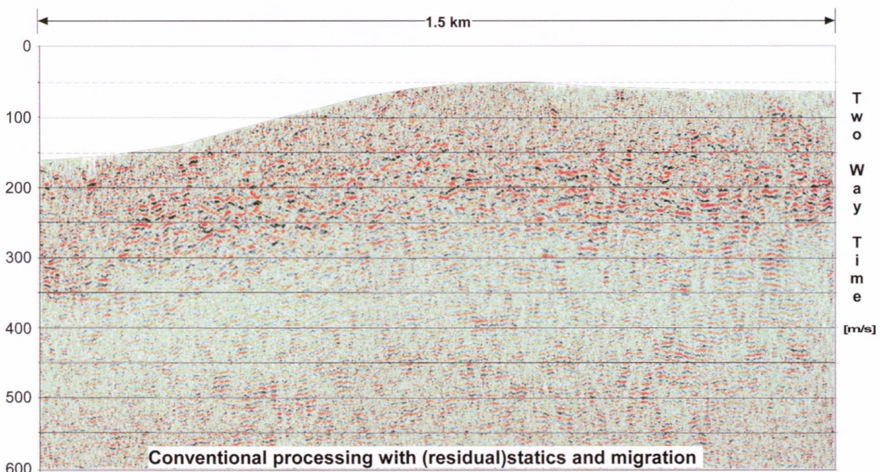
Fig. 3: Reflexionsseismisches Laufzeitprofil nach mehreren missbräuchlichen Durchläufen mit reststatischen Korrekturen und einer Migration.
