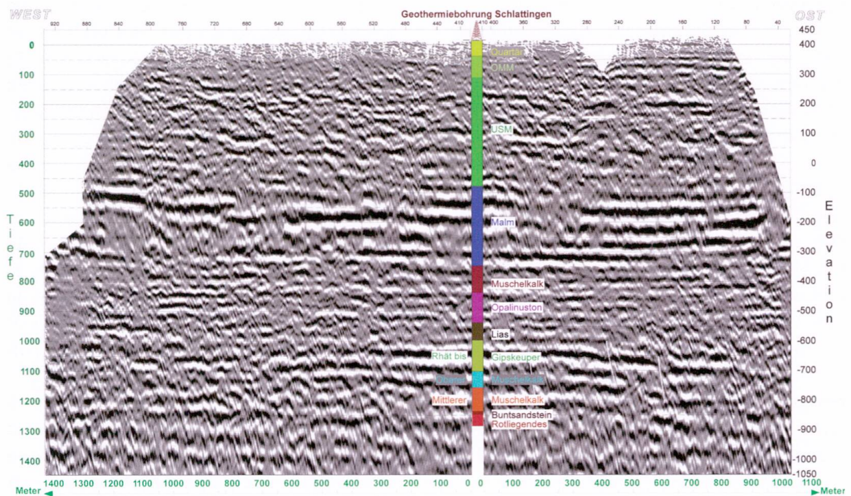
Fig. 1: Reflexionsseismisches Tiefenprofil über die Geothermiebohrung bei Schlattingen TG, erstellt mit einem Fallgewicht als seismische Quelle und registriert mit einer Registrierapparatur von 360 Datenkanälen, d. h. mit 360 aktiven Geophonstationen in Abständen von 2.7 m.
