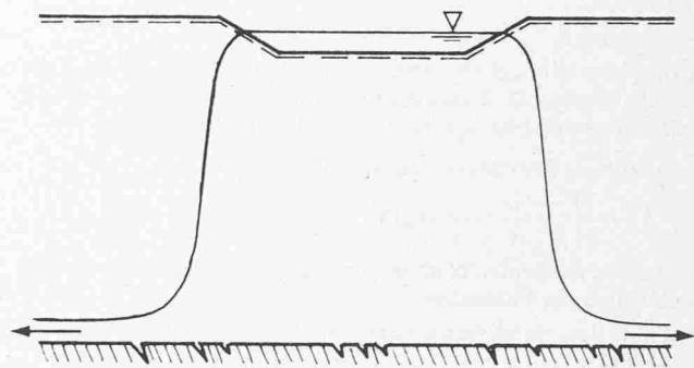
Bild 16. Freie Infiltration
