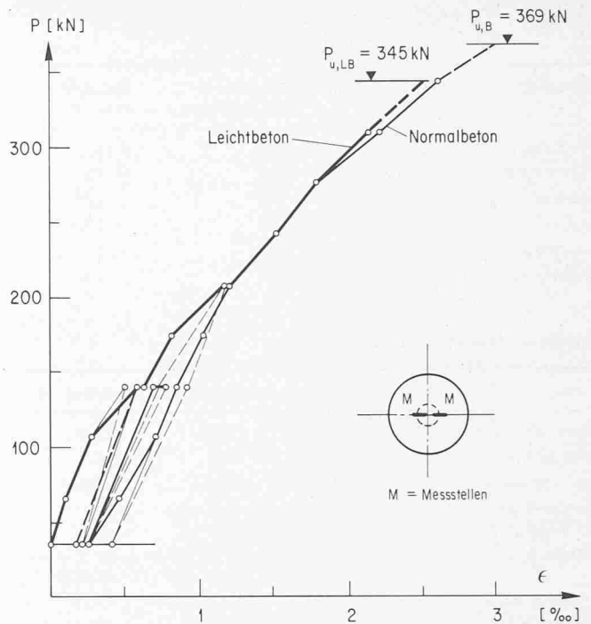
Bild 4. Last-Dehnungsdiagramme der Biegearmierung der obersten Lage
