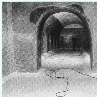
Wasserreservoir Muttenswald: Kombination von verschiedenen Sanierungs-Methoden: Injektionen gegen eindringendes Wasser und zur Verfestigung des Gewölbes, Auskleidung durch starre Abdichtung.
