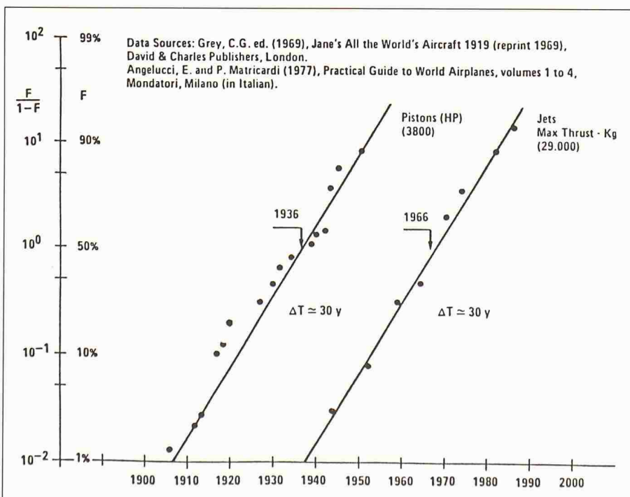
Bild 19. Wachstumspulse in der Leistung von Kolbenmotoren und Düsentriebwerken
