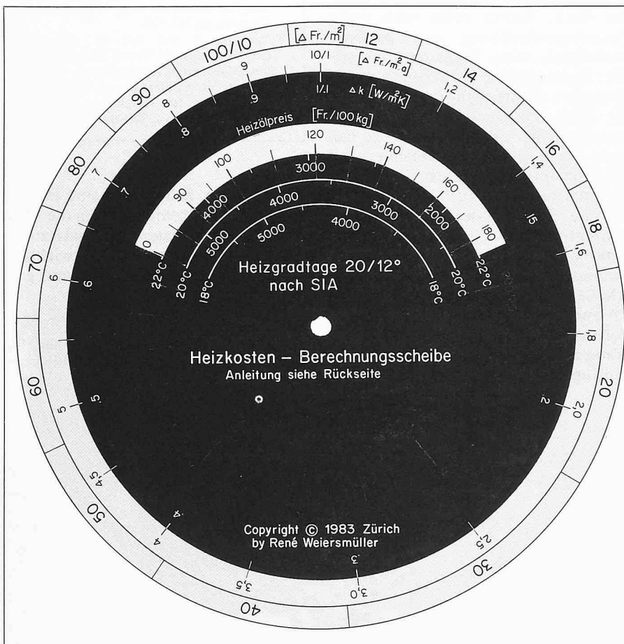
Bild 1. Vorderansicht der HK-Scheibe
