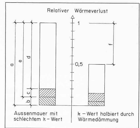
Bild 2. Relativer Wärmeverlust eines Bauteils bei k -Wertverminderung a Wärmeverlust aus k -Wert und Temperaturdifferenz b Gewinn aus Sonnenenergie durch direkte Bestrahlung c Anteilsmässiger Gewinn aus inneren Abwärmern und Sonneneinstrahlung durch Fenster d Durch Heizanlage zu deckender Verlust e Wärmeverlust für Optimierungen bzw. Wirtschaftlichkeitsberechnungen f Effektive Energieeinsparung an Heizanlage ohne Berücksichtigung des veränderten Teillastwirkungsgrades
