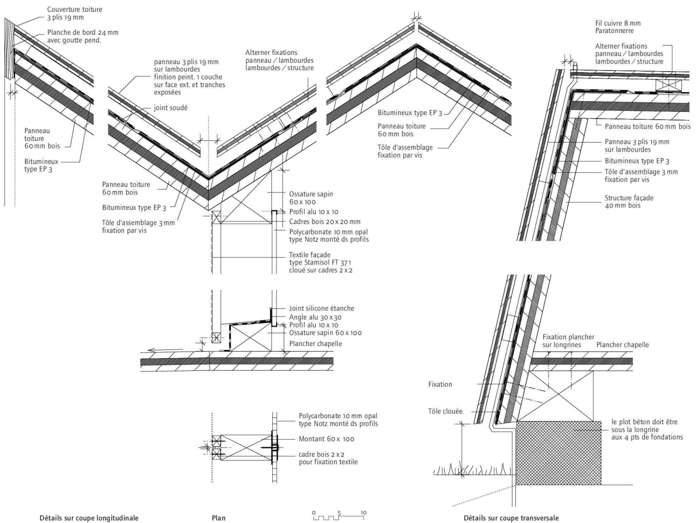
Détails sur coupe longitudinale
