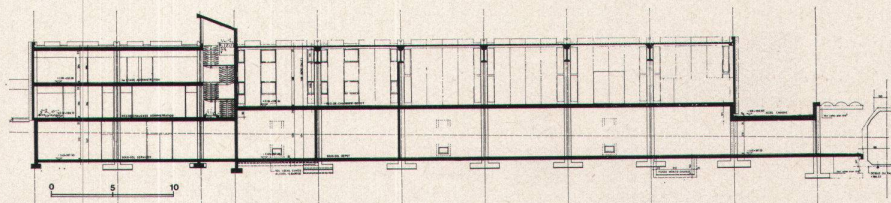
Schnitt
