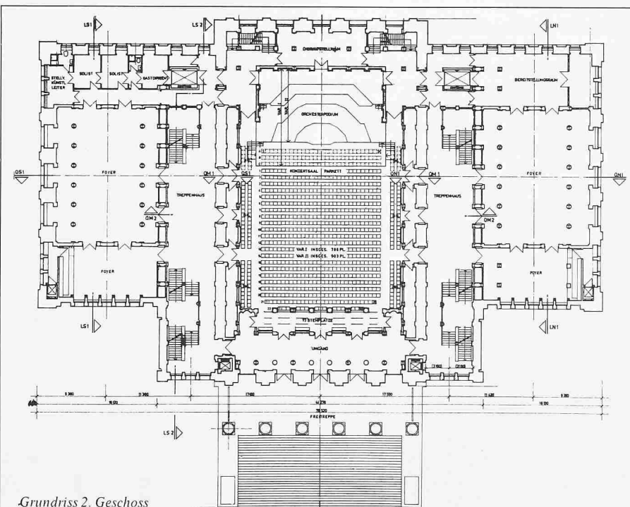
Grundriss 2. Geschoss
