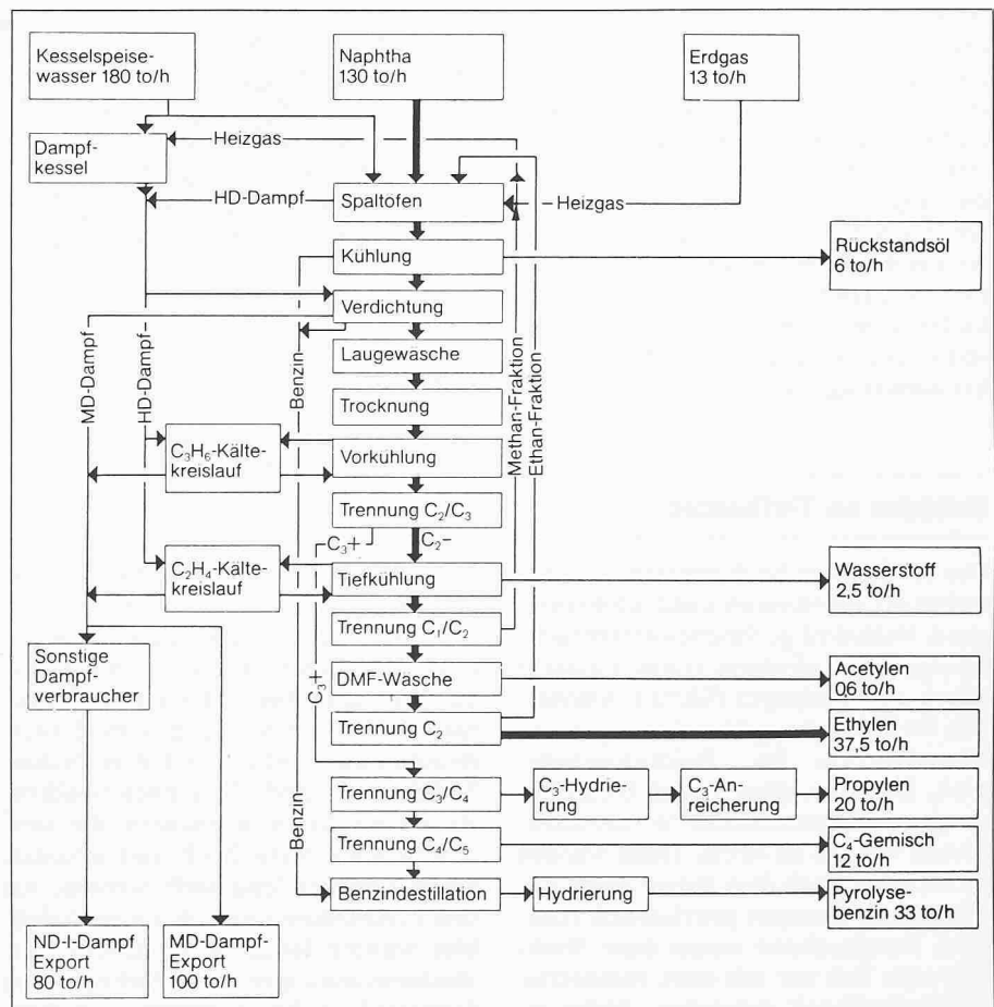
Steamcracker II: Vereinfachtes Fliesssche-ma. Stand: November 1980
