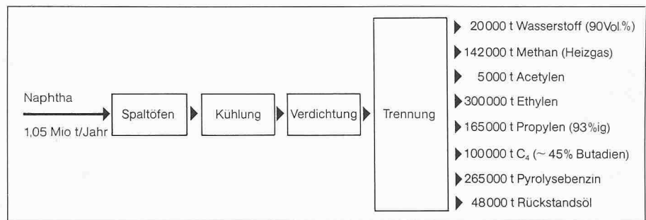
Steamcracker II: Stark vereinfachtes Fliesssche-ma. Stand: November 1980
