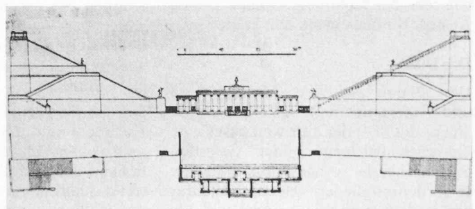
Bild 2. Panathenäisches Stadion in Athen. Grundriss und Schnitt (Foto eines Originalplans). Eine langgestreckte Tribünenanlage umgibt die Kampfbahn, die sich als unzureichend erwies
