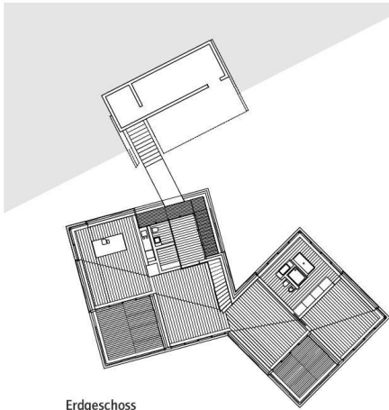
Erdgeschoss
