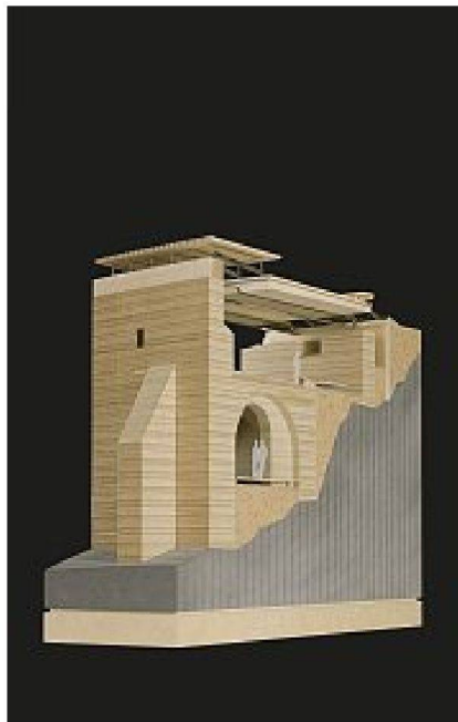
Schnittmodell Revitalisierung Altane Stift Altenburg, Konstruktion der neuen Überdachung.
