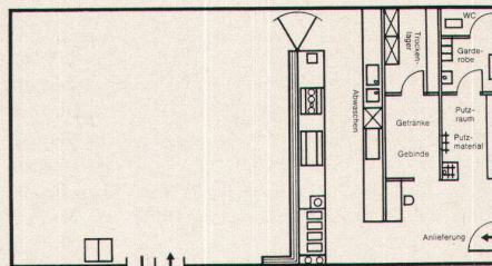
Planungsbeispiel eines Personalrestaurants mit Warmanlieferung
