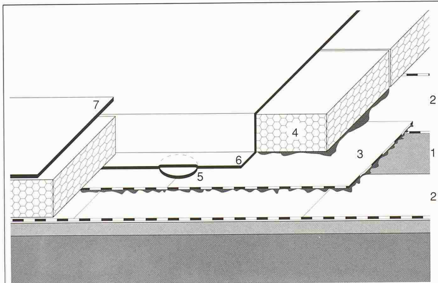
1 Unterkonstruktion im Gefälle 2 Bituminöse Dampfsperre, lose verlegt oder vollflächig aufgeklebt 3 Sarnacombivap-Streifen, als nicht unterwanderbare Wasserbarriere aufgeklebt oder aufgeflämmt 4 Wärmedämmschicht (z.B. Sarnatherm), eine Plattenreihe als Anschlag für die Ausführung der Abschottung aufgeklebt 5 Sarnafil G 469-10-Rondelle über den Sarnacombivap-Bahnenstössen 6 Sarnafil-Abdichtung, mit dem Sarnacombivap-Streifen verschweisst 7 Sarnafil-Abdichtungen, miteinander verschweisst
