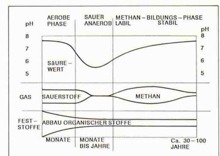
Bild 2. Die Entwicklungsphasen einer Reaktordeponie
