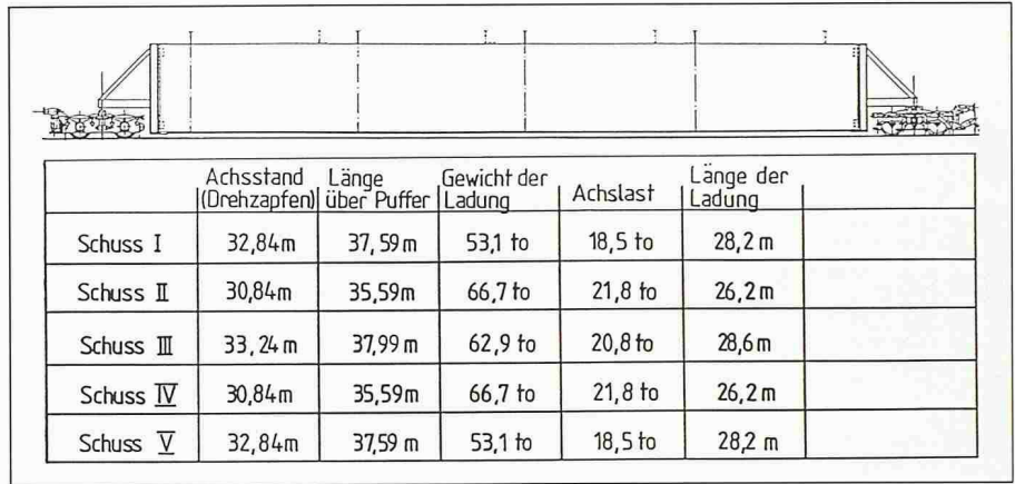
Bild 7. Transportkonzept mit Abmessungen und Gewichten. Die Trägerunterkante befindet sich 17 cm über den Schienen
