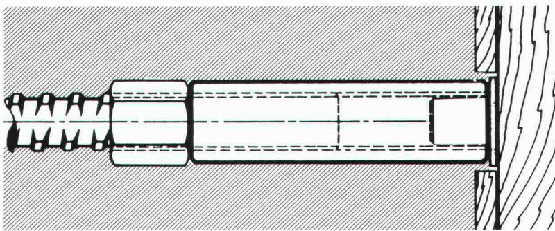
Gewi-Muffenstoss
