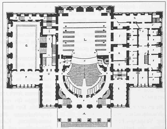
Schauspielhaus, ursprünglicher Erdgeschossgrundriss, Zuschauerraum, Bühne
