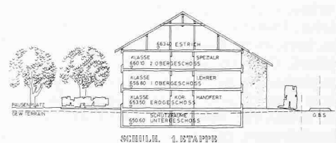
Schnitt 1:900
