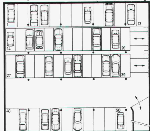
50 Parkplätze mit VARIO-AUTOPARKER Gewinn 20 Plätze resp. 66 % bei gleicher Fläche und gleichem Bauvolumen.
