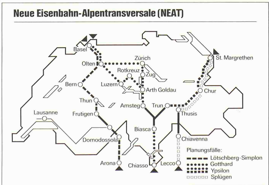
Bild 1. Kartographisches Schema der untersuchten NEAT-Planungsfälle
